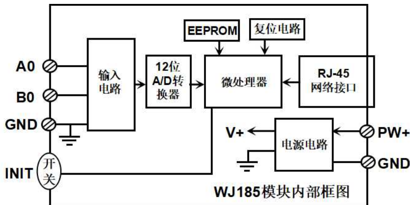
图2 WJ185 模块内部框图
